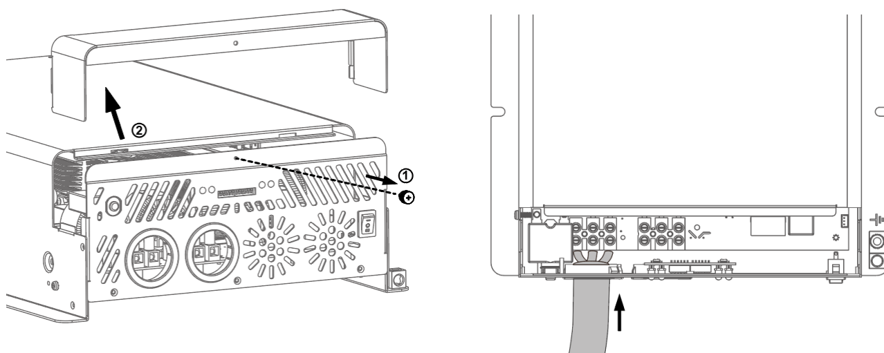
Fig. 10 : SC-3000 Installation
