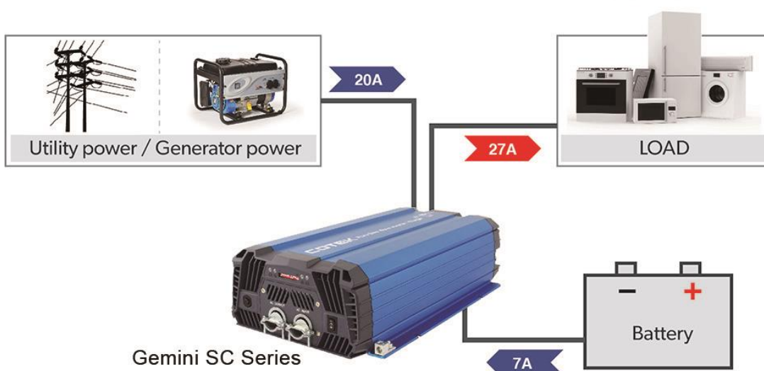
Fig. 21 : Generator Function
