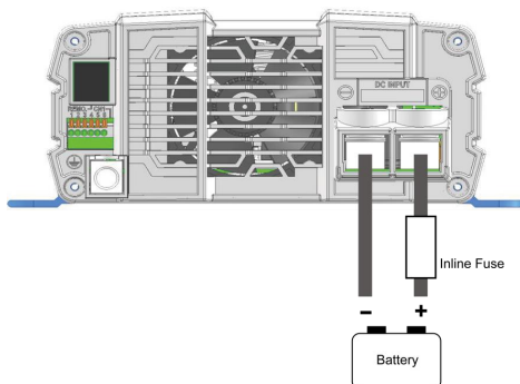
Schéma 18 – Connexion batterie-onduleur
