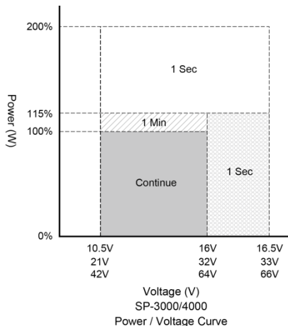
Schéma 3 – SP-3000~SP-4000 Puissance en sortie / Tension d'alimentation
