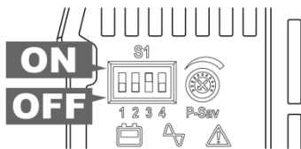
Schéma 10 – Interrupteurs DIP
