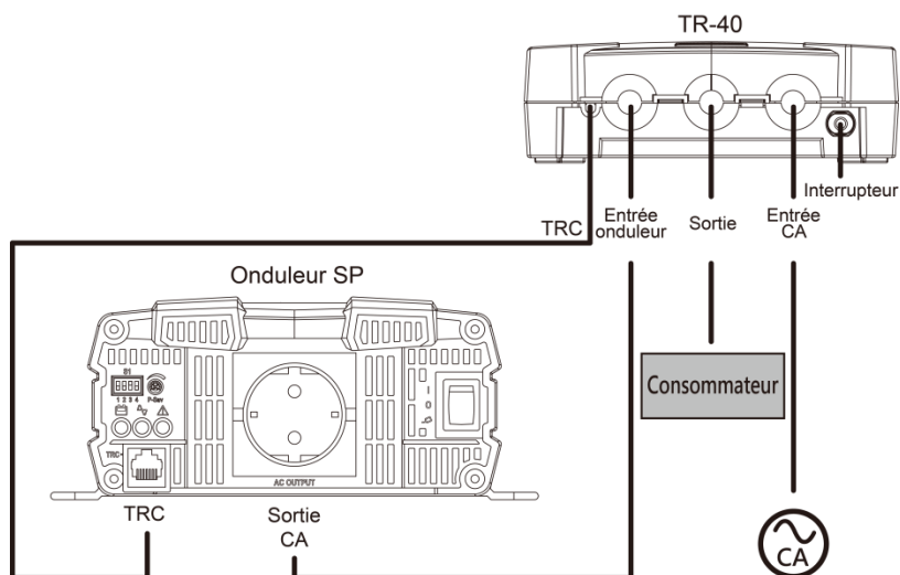
Schéma 11 – Connexions onduleur SP / TR-40
