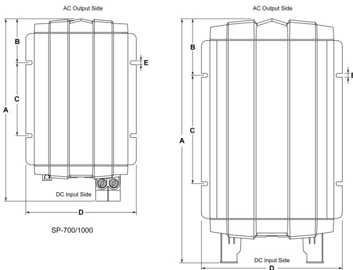
Schéma 5 – Onduleurs série SP (vue de dessus)
